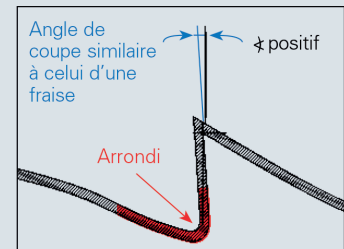
Profil de la lime Multifile
